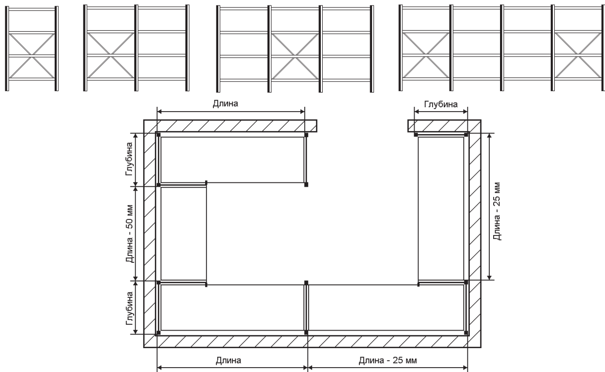
Комбинации стеллажей
